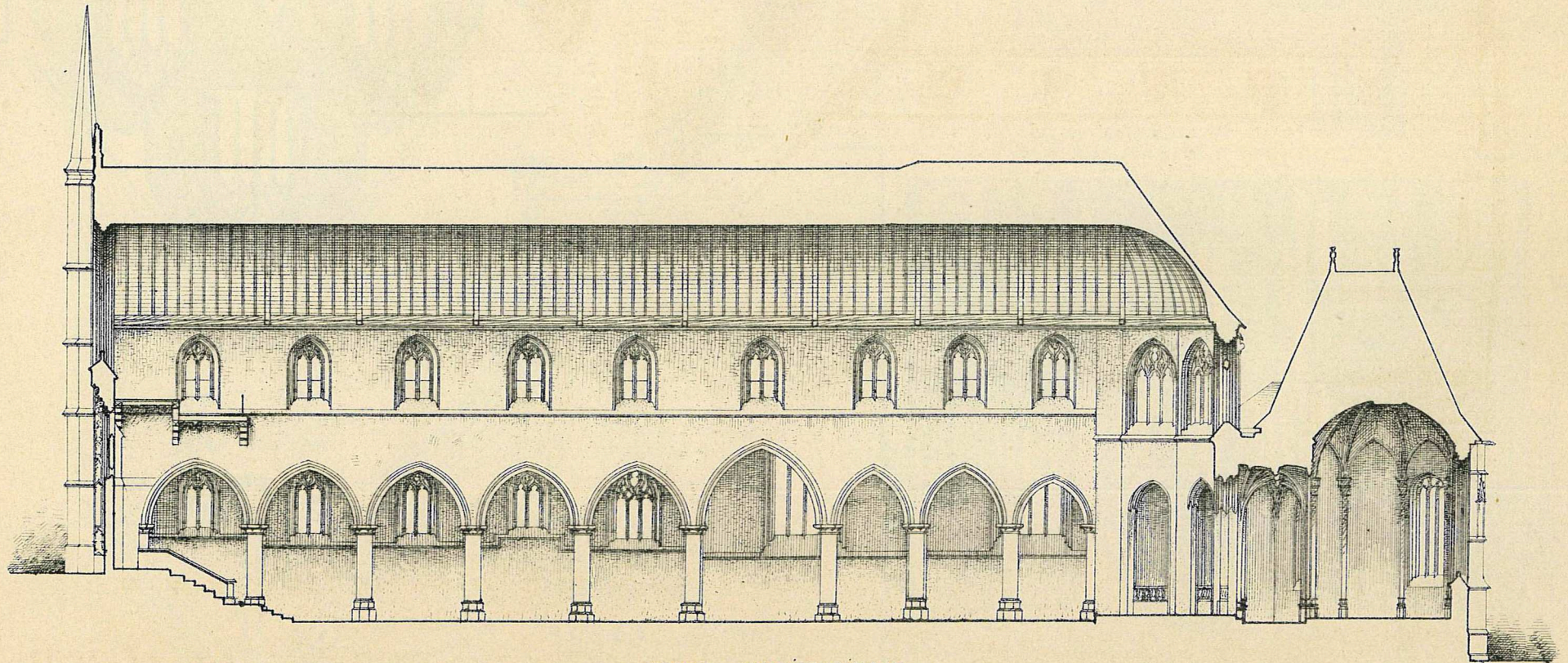
COUPE LONGITUDINALE.
