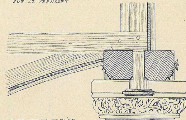
CORBELS SERVANT DE POINT D'APPUI AUX FOUTRES PANNES.
