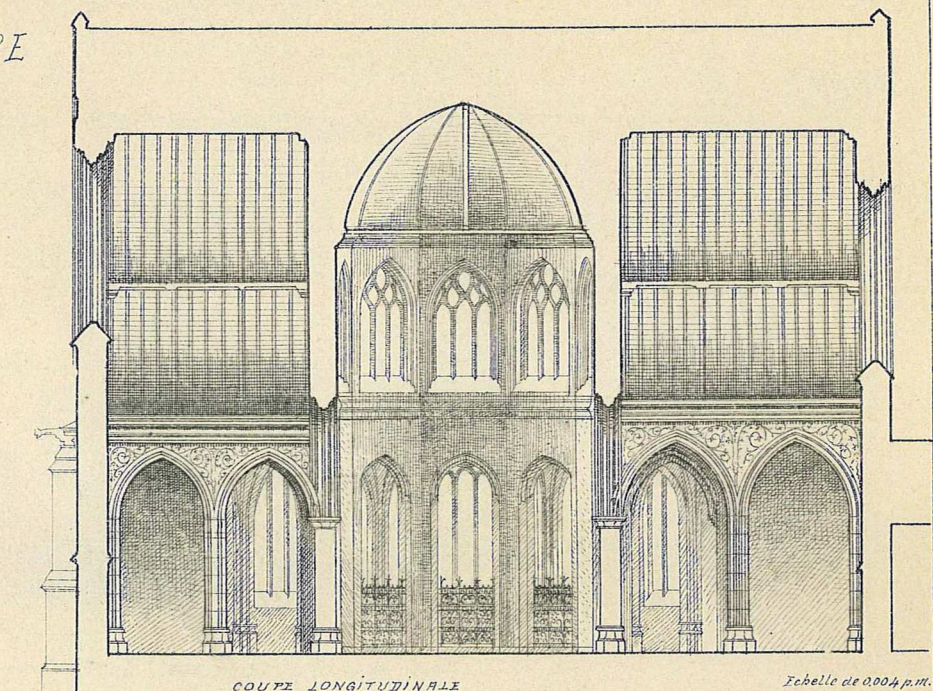
COUPE LONGITUDINALE SUR LE TRANSEPT
