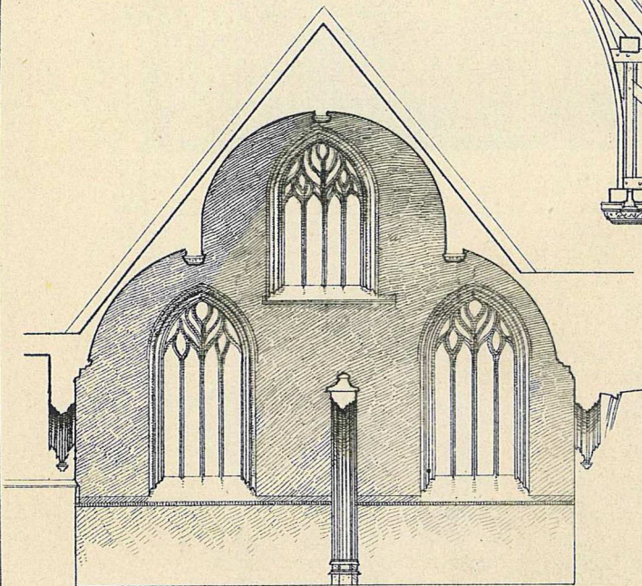
COUPE SUR UN DES BRAS DU TRANSEPT. Echelle de 0.004 p.m.
